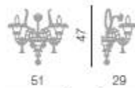
Zeus parete 2L L 51 cm - H 47 cm - SP 29 cm 2 x E14 40W
