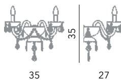
Parigi parete 2L L 35 cm - H 35 cm - SP 27 cm 2 x E14 40W
