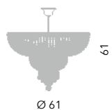
Asburgo sospensione Ø 60 cm Ø 61 cm - H 61 cm 8 x E14 40W
