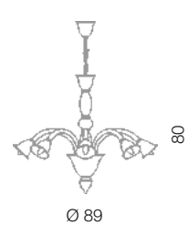
Artemide lampadario 8L BB Ø 89 cm - H 80 cm 8 x E14 40W
