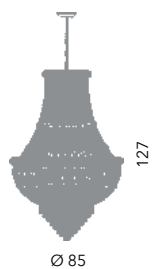
Tokyo lampadario Impero Ø 80 cm Ø 85 cm - H 127 cm 15 x E14 40W
