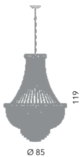
Borbone lampadario Impero Ø 80 cm Ø 85 cm - H 119 cm 15 x E14 40W
