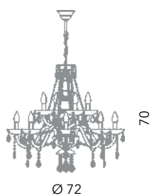
Parigi lampadario 8+4L Ø 72 cm - H 70 cm 12 x E14 40W
