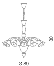
Artemide lampadario 12L BB Ø 89 cm - H 80 cm 12 x E14 40W
