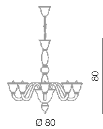
Artemide lampadario 8L Ø 80 cm - H 80 cm 8 x E14 40W
