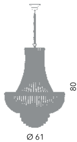
Monaco sospensione Ø 60 cm Ø 61 cm - H 80 cm 9 x E14 40W
