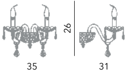
Zurigoparete 2L L 35 cm - H 26 cm - SP 31 cm 2 x E14 40W
