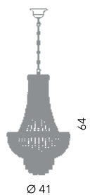
Monaco sospensione Ø 40 cm Ø 41 cm - H 64 cm 6 x E14 40W
