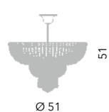
Asburgo sospensione Ø 50 cm Ø 51 cm - H 51 cm 6 x E14 40W
