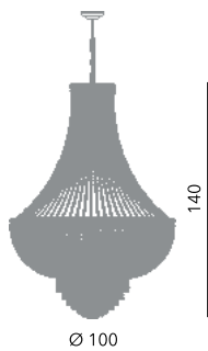
Monaco sospensione Ø 100 cm Ø 100 cm - H 140 cm 18 x E14 40W
