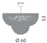
Monaco sospensione Ø 60 cm Ø 60 cm - H 53 cm 8 x E14 40W
