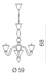
Artemide lampadario 4L Ø 59 cm - H 68 cm 4 x E14 40W
