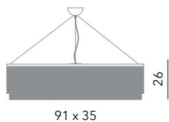
Pioggia lampadario ovale 6L L 91 x 35 cm - H 26 cm 6 x G9 60W
