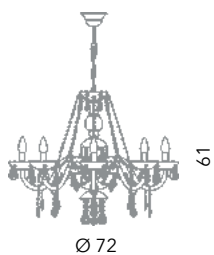
Parigi lampadario 8L Ø 72 cm - H 61 cm 8 x E14 40W
