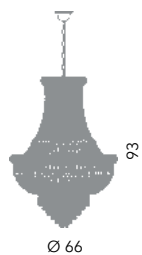
Tokyo lampadario Impero Ø 60 cm Ø 66 cm - H 93 cm 9 x E14 40W
