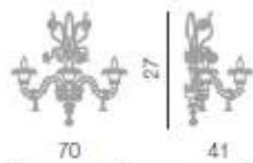
Zeus parete 3L L 70 cm - H 27 cm - SP 41 cm 3 x E14 40W
