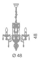
Madrid lampadario 3L Ø 48 cm - H 48 c 3 x E14 40W
