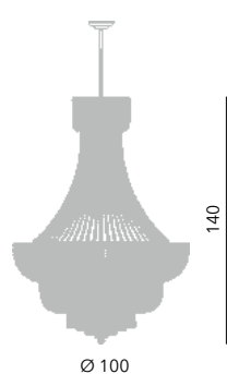
Asburgo lampadario Impero Ø 100 cm Ø 100 cm - H 140 cm 18 x E14 40W
