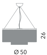
Pioggia lampadario rotondo 6L Ø 50 cm - H 26 cm 6 x G9 60W
