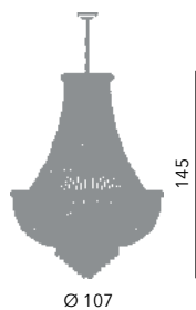
Tokyo lampadario Impero Ø 100 cm Ø 107 cm - H 145 cm 18 x E14 40W
