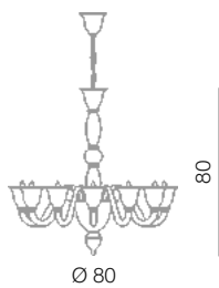
Artemide lampadario 12L Ø 80 cm - H 80 cm 12 x E14 40W
