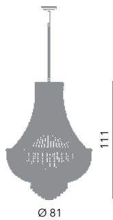
Stuart lampadario Impero Ø 80 cm Ø 81 cm - H 111 cm 15 x E14 40W
