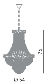
Borbone lampadario Impero Ø 50 cm Ø 54 cm - H 76 cm 7 x E14 40W
