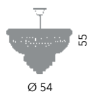
Tokyo sospensione Ø 50 cm Ø 54 cm - H 55 cm 6 x E14 40W
