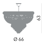
Tokyo sospensione Ø 60 cm Ø 66 cm - H 63 cm 8 x E14 40W
