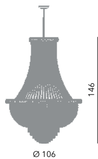
Borbone lampadario Impero Ø 100 cm Ø 106 cm - H 146 cm 18 x E14 40W
