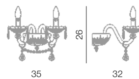
Madrid parete 2L L 35 cm - H 26 cm - SP 32 cm 2 x E14 40W
