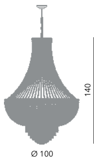
Stuart lampadario Impero Ø 100 cm Ø 100 cm - H 140 cm 18 x E14 40W
