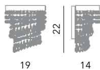
Mosca parete 2L L 19 cm - H 22 cm - SP 14 cm 2 x E14 40W
